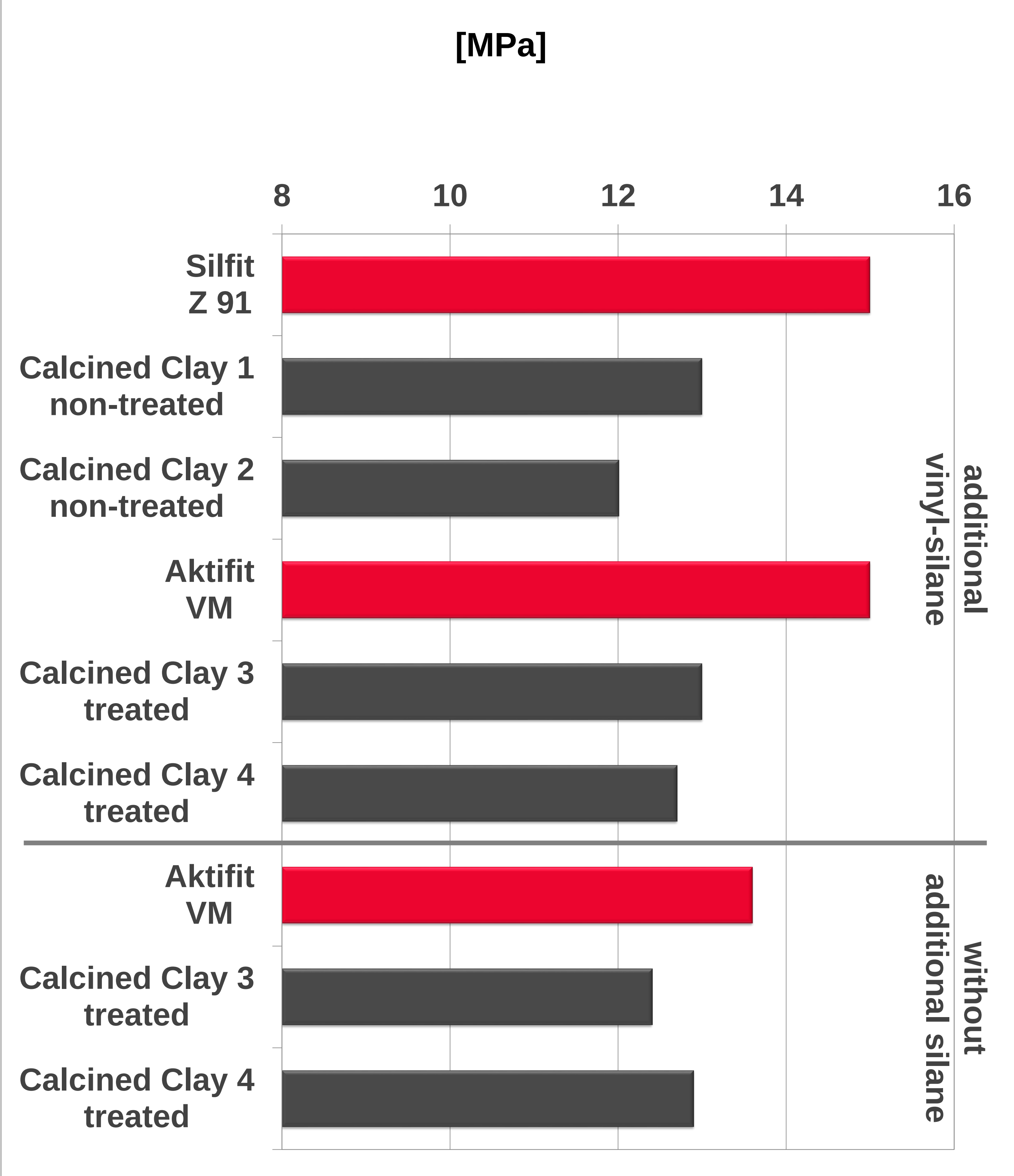
Tensile Strength
